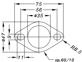
VISTA DA "B" Flangia tipo "45A"
