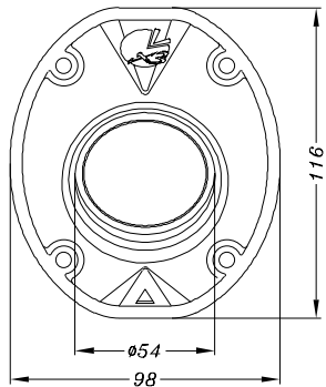
VISTA DA "A"
