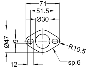
Vista "B" Flangia "43D"
