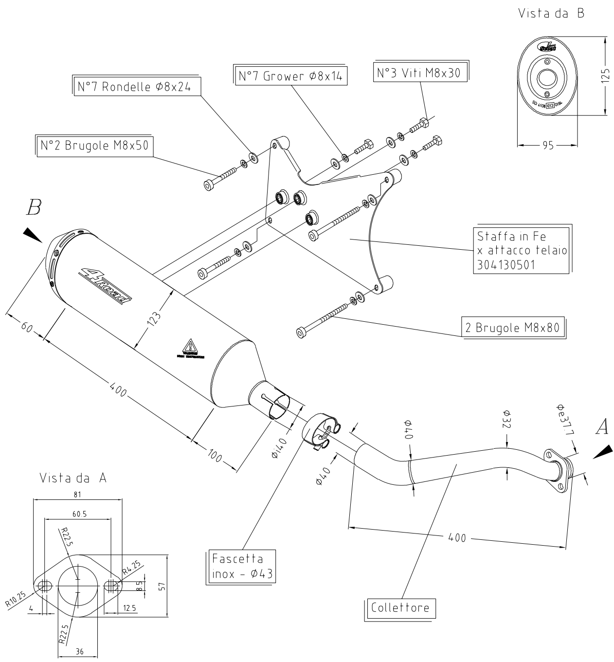
ART. 4130 Silenziatore << 4 ROAD >> per HONDA FORESIGHT 250 (fino al '99)
