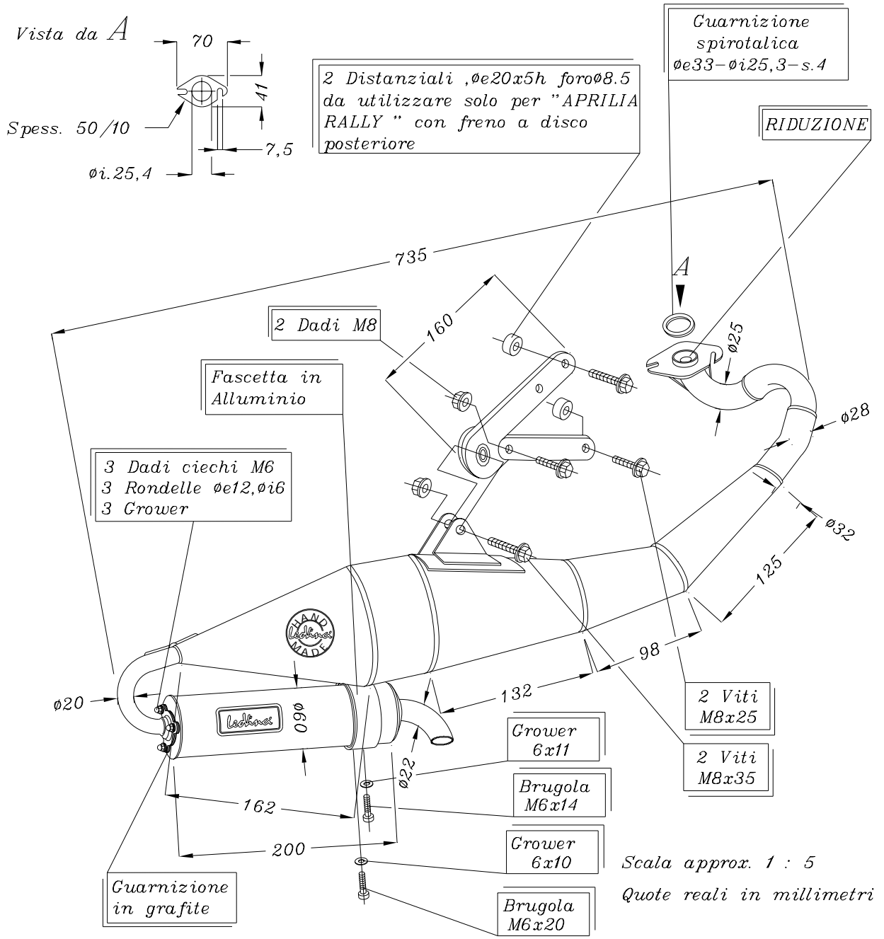
ART. 4277 Silenziatore HANDE MADE "RS" per APRILIA RALLY con silenziatore in inox.
